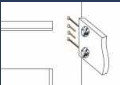
detail spojů konstrukce postele
